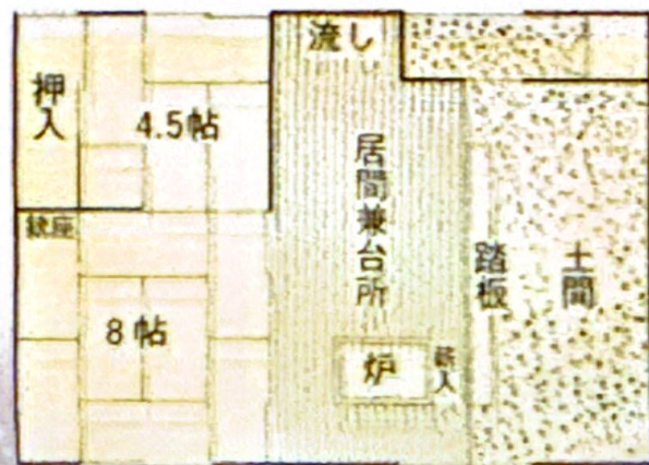
屯田兵屋平面図
